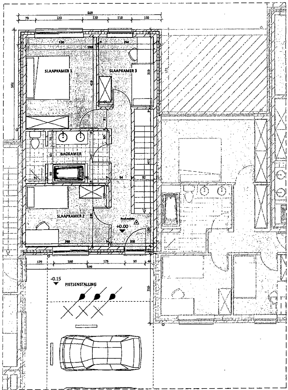
WONING 03 - GELIJKVLOERS
